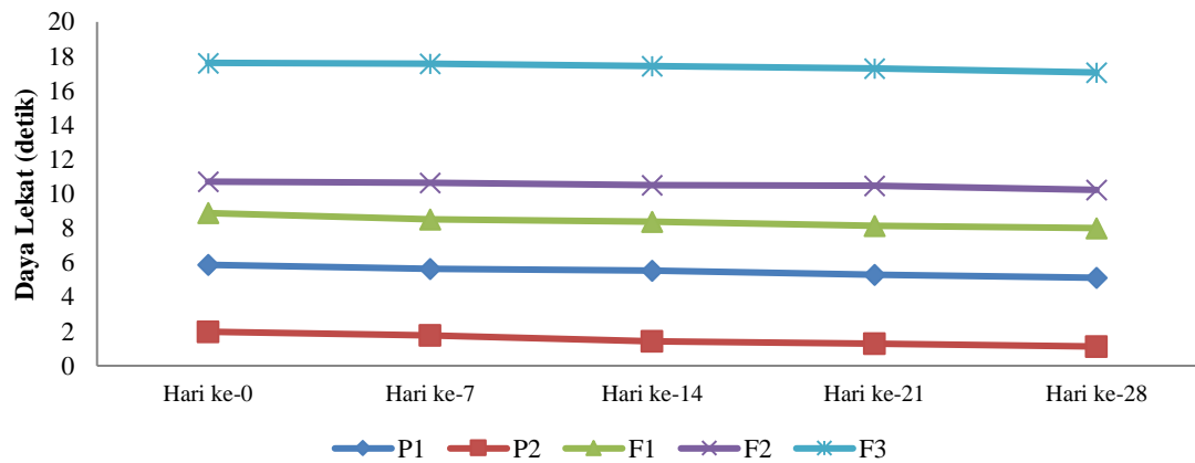
Gambar 6. Grafik Hubungan Daya Lekat dan Waktu Penyimpanan
