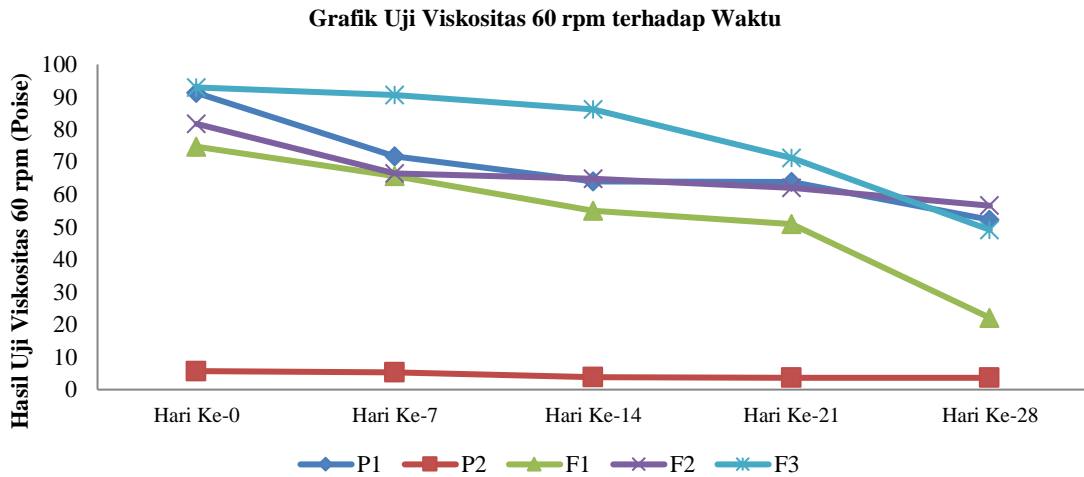
Gambar 4. Grafik Hubungan Viskositas 60 rpm dan Waktu Penyimpanan
