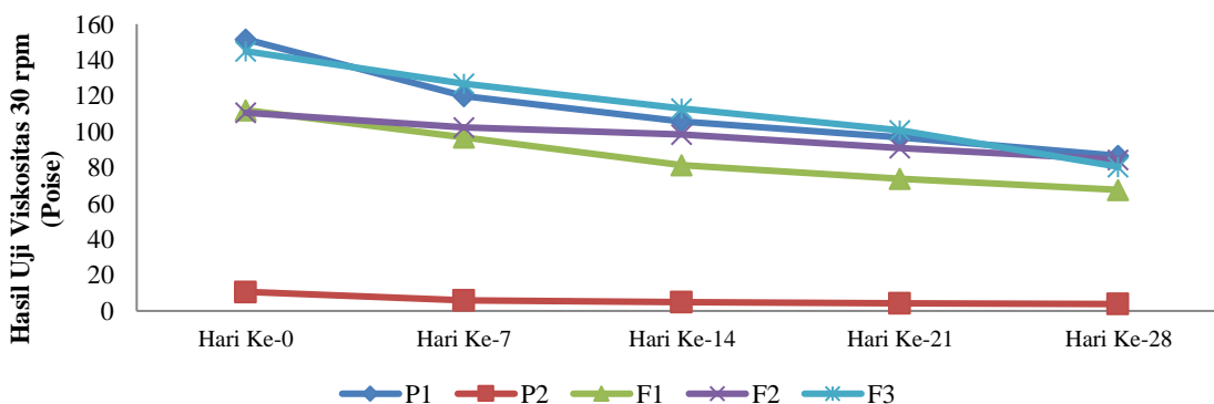
Grafik Uji Viskositas 30 rpm terhadap Waktu
